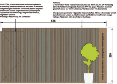
ANSICHT WANDVERKLEIDUNG STIRNSEITE NEU GEGENSEITE
